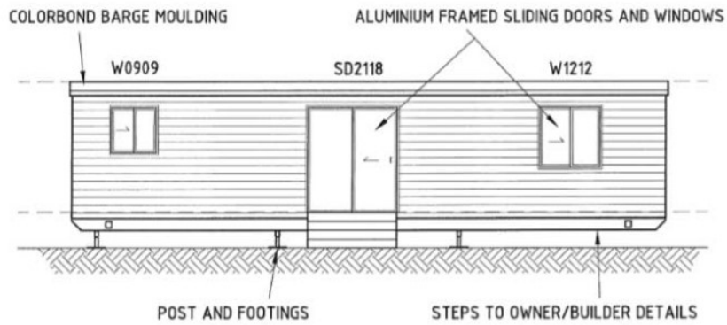
ELEVATION - A 1:100
