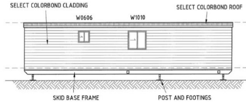
ELEVATION - B 1:100
