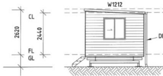
ELEVATION - D 1:100
