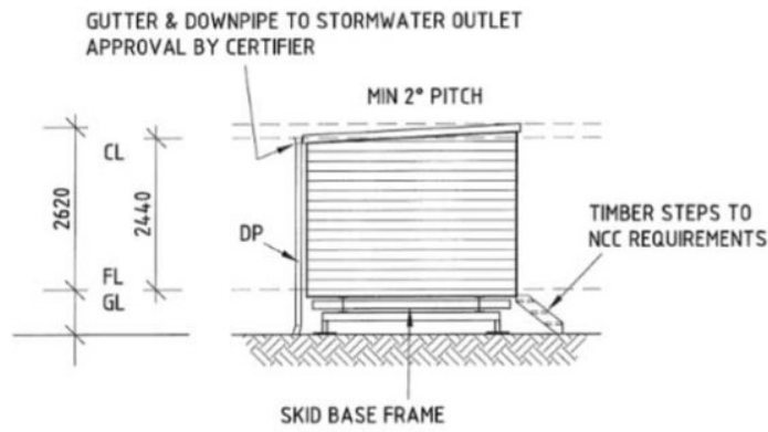
ELEVATION - C 1:100
